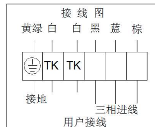
接线图 (默认为不带热保护器)
