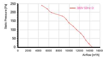
性能曲线
