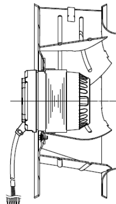
轴水平安装
