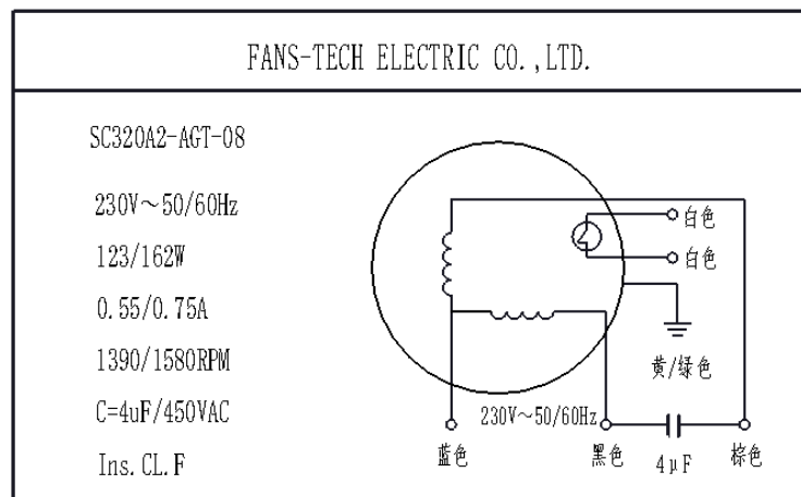
铭牌
