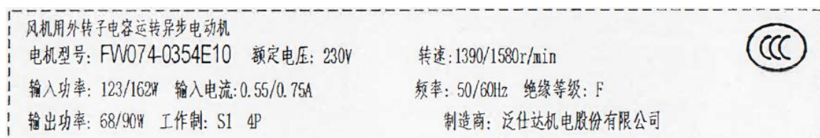
丝印铭牌
